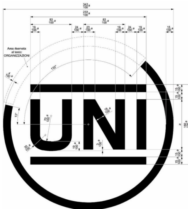
Versione quotata
